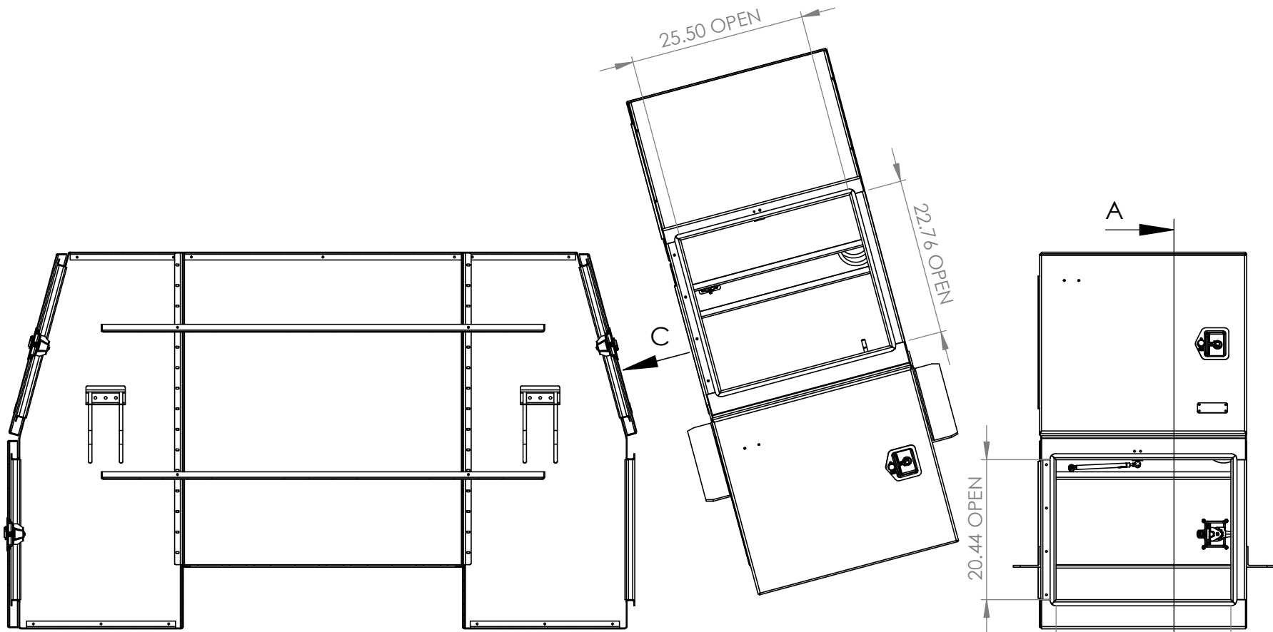
SECTION A-A
